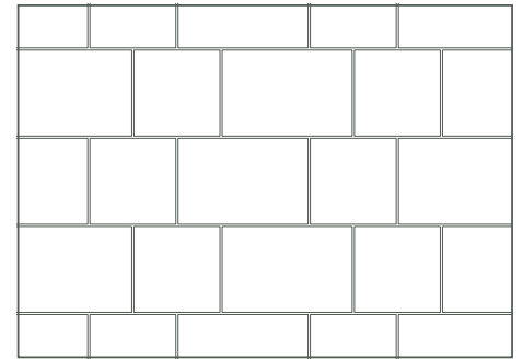
Patrón: rompe juntas con dos formatos Formatos: 16 x 16 cm · 16 x 24 cm 40 x 40 cm · 40 x 60 cm
