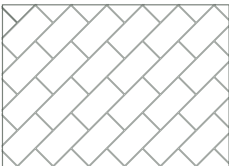
Patrón: rompe juntas a 45° Formatos: 10 x 20 cm ó 20 x 40 cm
