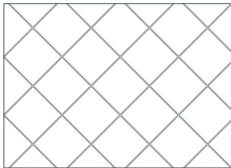
Patrón: junta seguida a 45° Formatos: 16 x 16 cm ó 40 x 40 cm
